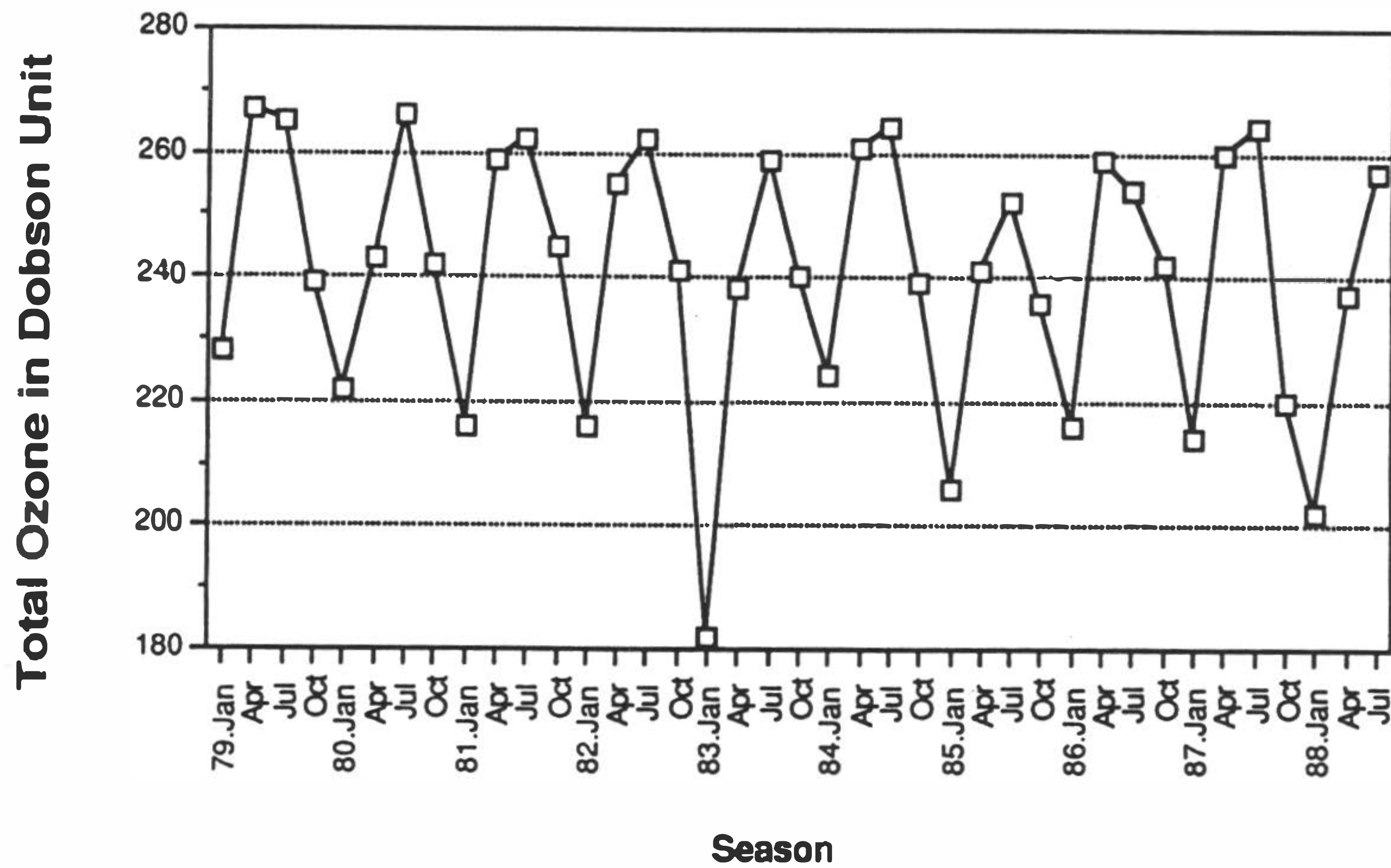
Fig. 2. Ozone trends on the 20N-30N latitude band, 1979-1988.
